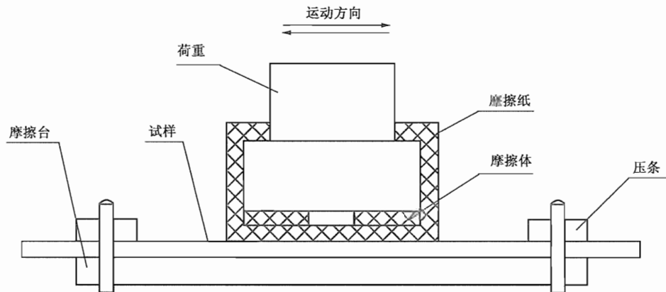
图 1 摩擦试验机
